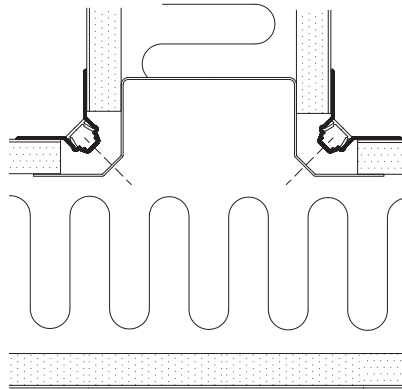
T-connection
