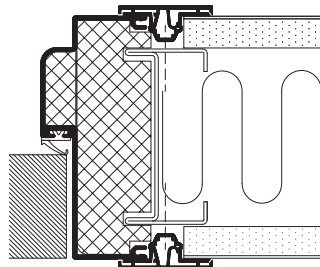
Solid door
